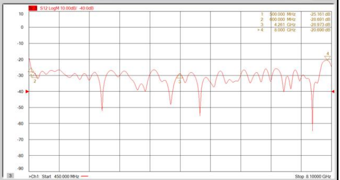
图2: 隔离度
