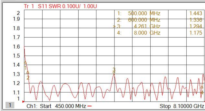
图1:输入驻波
