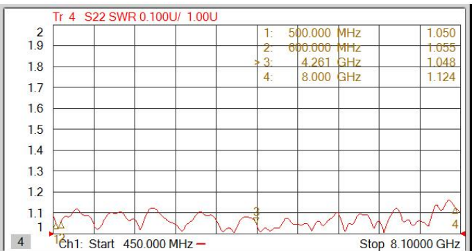
图4: 输出驻波
